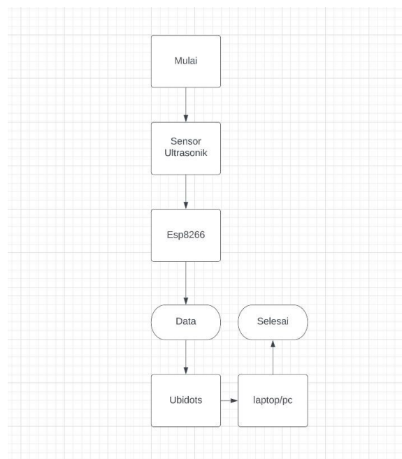
Gambar 3. Diagram alir sistem
